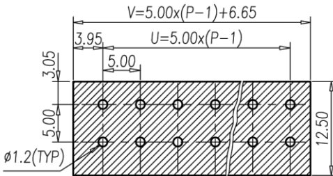
P.C.B. LAYOUT(REF)
