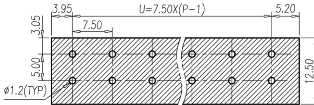
P.C.B. LAYOUT(REF)
